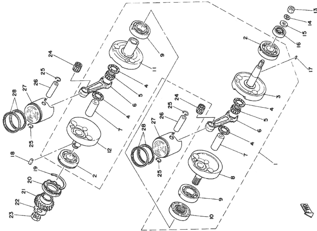
Fig. 4 CRANK - PISTON (2)
